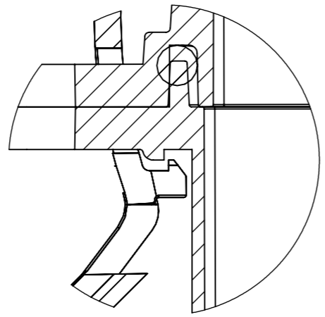
DETAIL D SCALA 2 : 1
