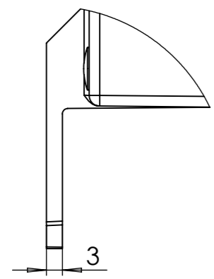
DETTAGLIO H SPESSORE PUNTI DI ATTACCO REV3 SCALA 1 : 1
